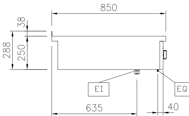
Zij aanzicht
