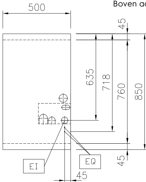
Boven aanzicht
